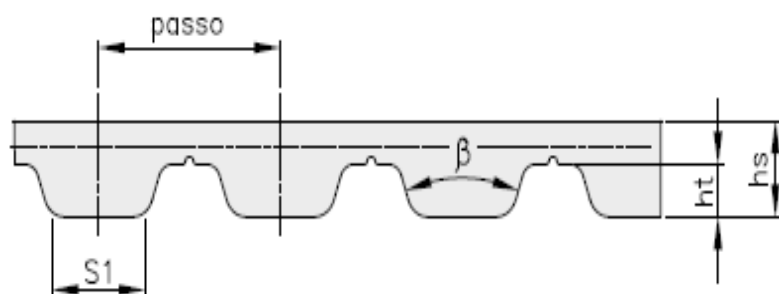
DIMENSIONS
